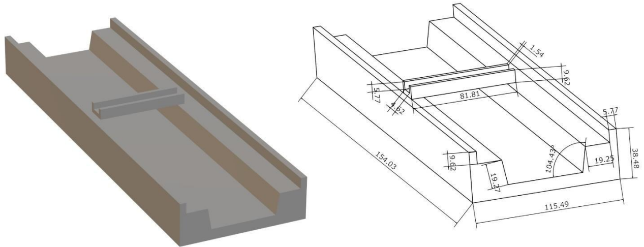
Figura 2. Modelo 3D de un canal de agua con un puente que la atraviesa de forma transversal (izquierda). Medidas del sistema dadas en unidades \times 10^{-1}m (derecha).
